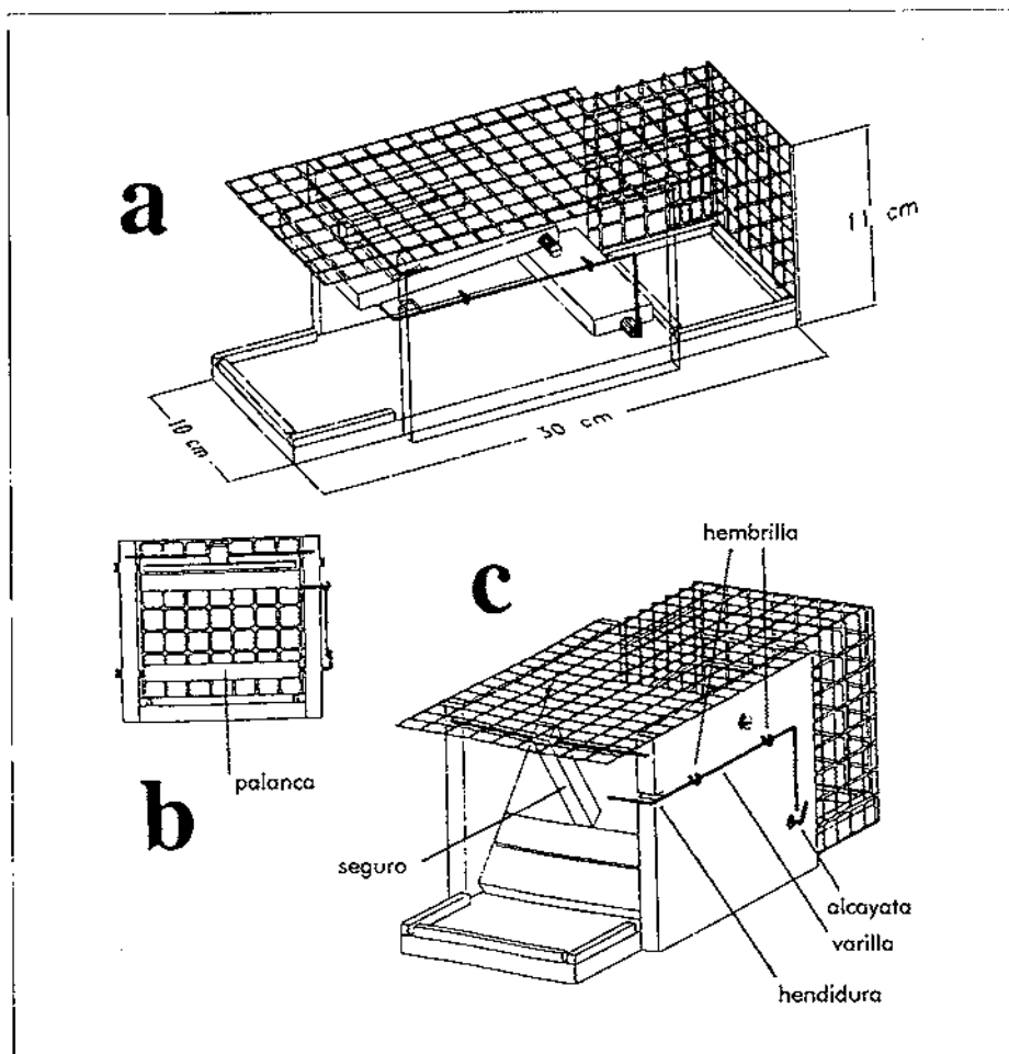
Figura 1. Diseño y medidas de la trampa automática: a) vista lateral en posición activada; b) vista frontal con mecanismo activado; c) trampa disparada.
